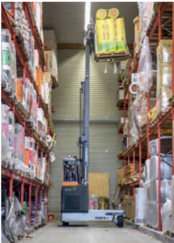
Vierwegzijlader met energie-efficiënte dieselaandrijving Vierwegestapler mit energieeffizientem Dieselantrieb
